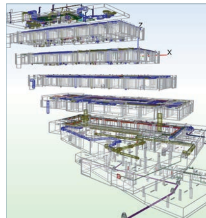
Figura 2. Maqueta en 3D por BIM.
