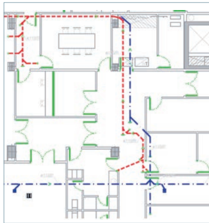
Figura 5. Plano de redes de saneamiento.
